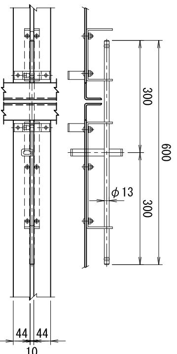
正面図 (S=1/20)
