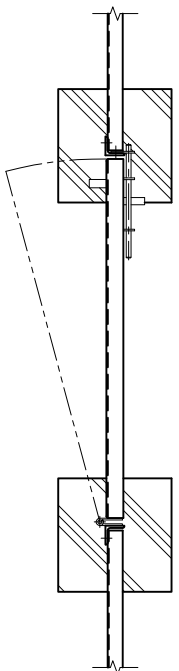
平面図 (S=1/20)
