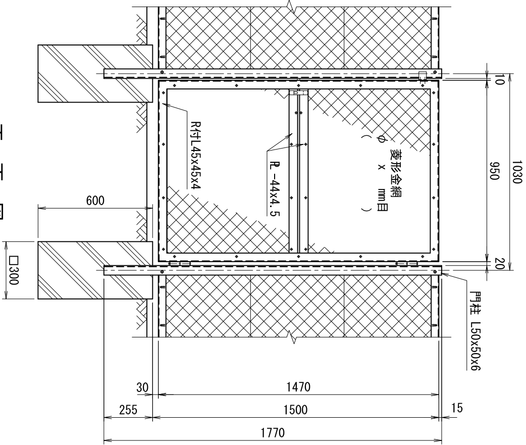
平面図 (S=1/20)
