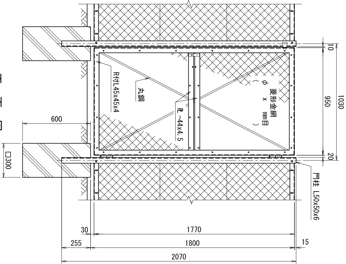
平面図 (S=1/20)
