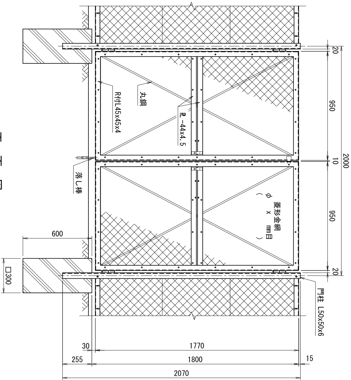
平面図 (S=1/20)
