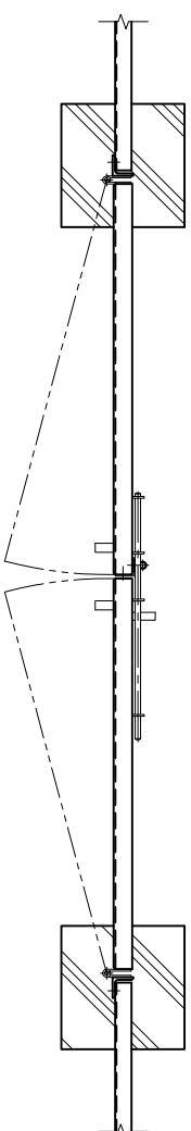
平面図 (S=1/20)
