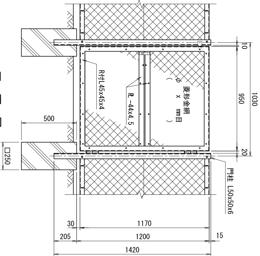
正面図 (S=1/20)
