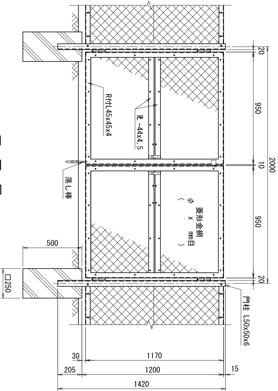
正面図 (S=1/20)
