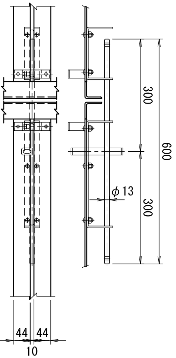
正面図 (S=1/20)
